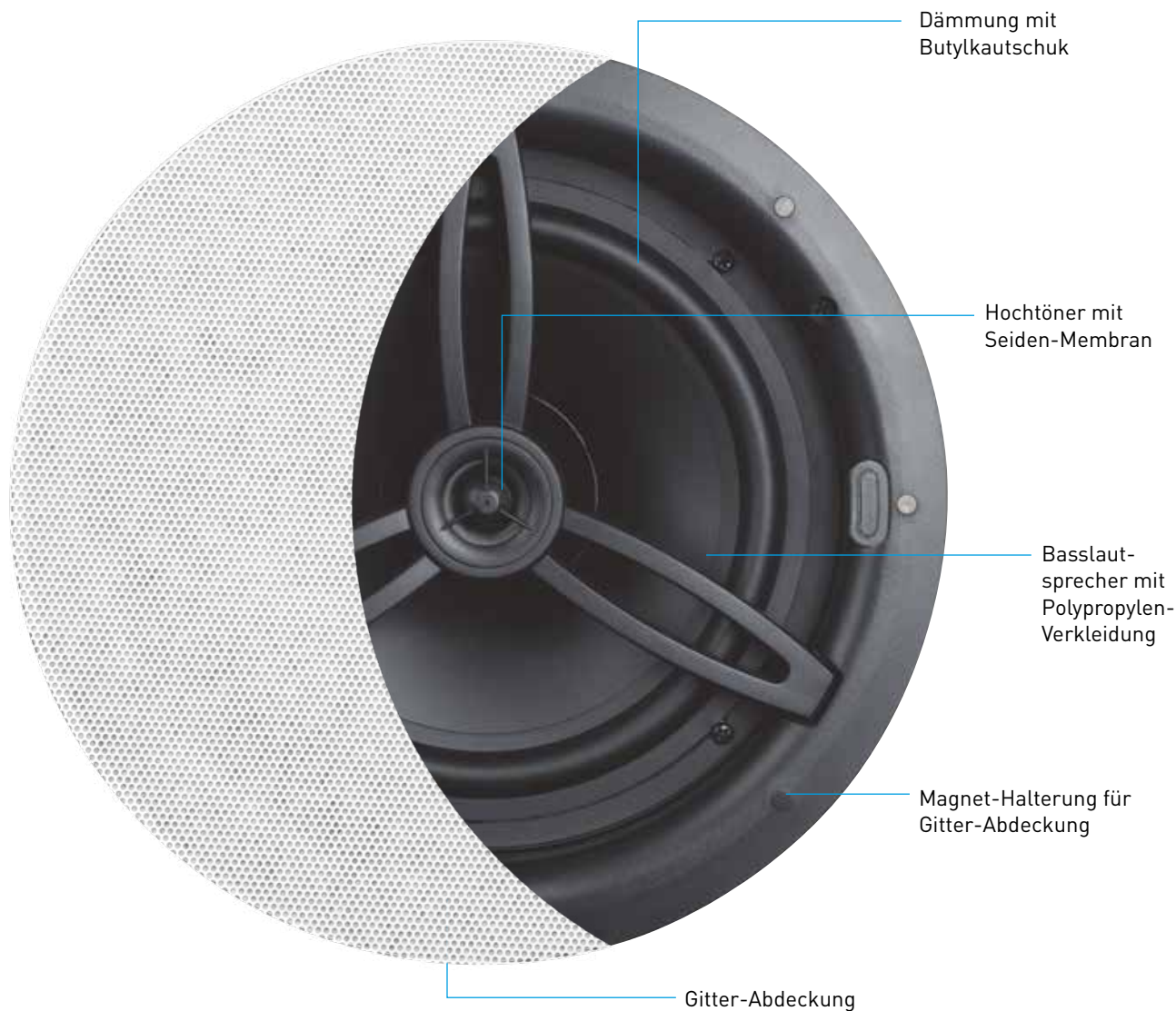
Deckenlautsprecher
