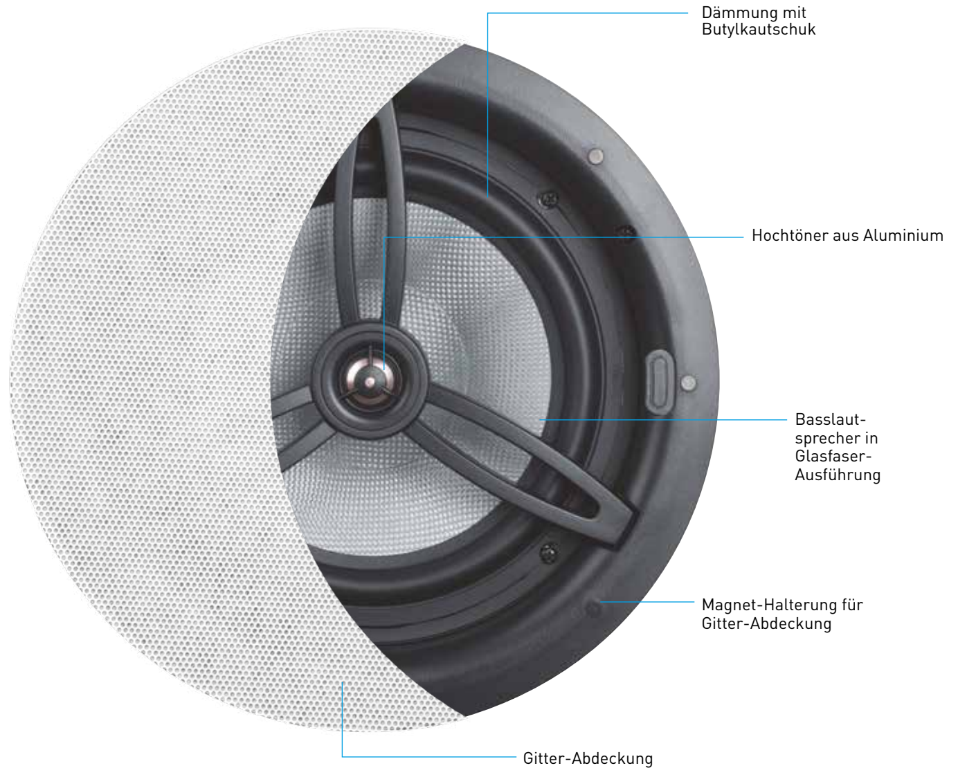
Deckenlautsprecher
