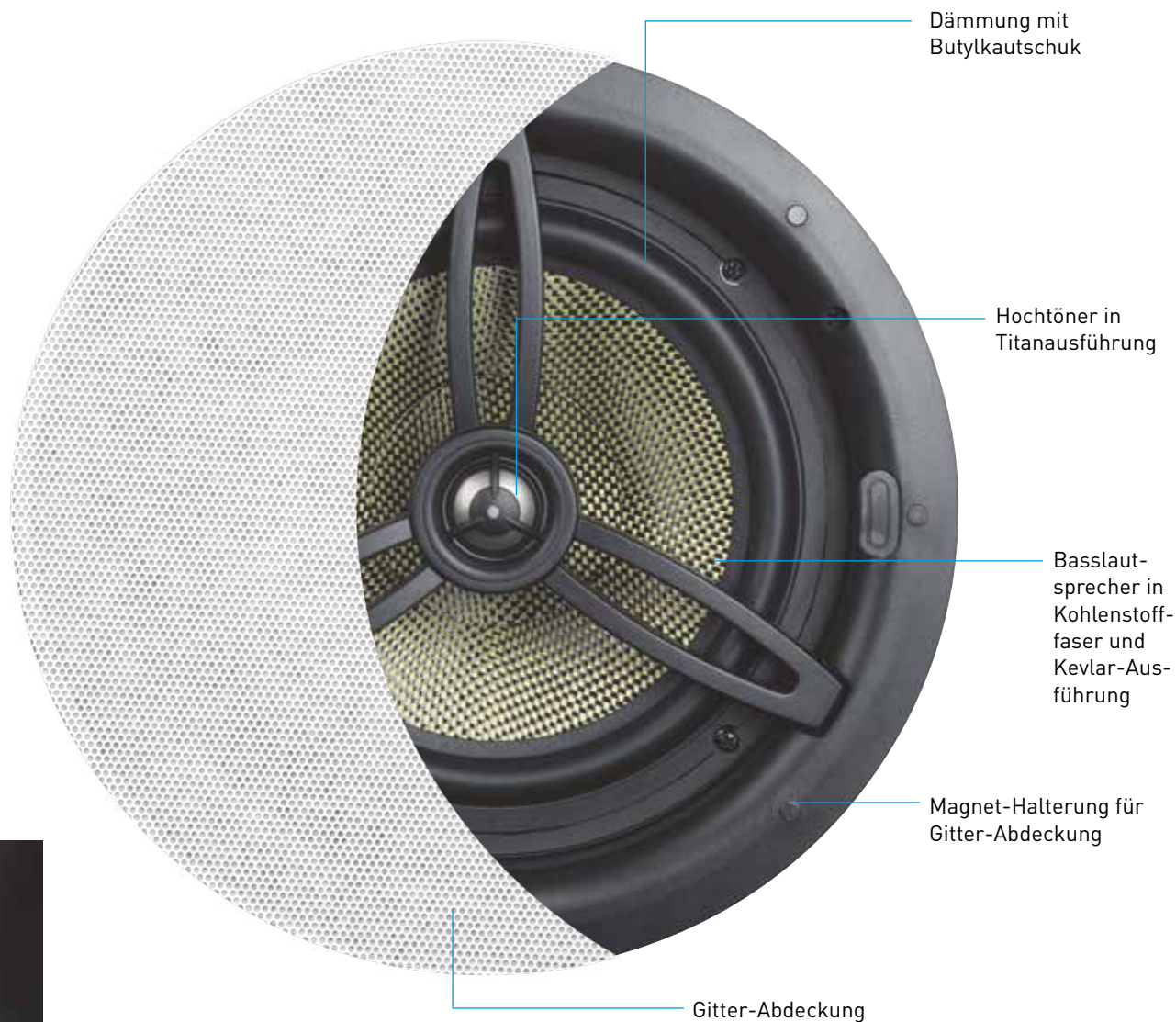
Deckenlautsprecher
